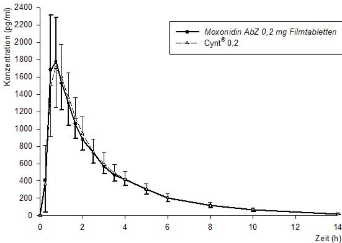
Abb. 1: Mittelwerte und Standardabweichungen der Plasmakonzentration von Moxonidin nach Einmalgabe von 1 Filmtabletten Moxonidin AbZ 0,2 mg Filmtabletten bzw. Cynt® 0,2.
