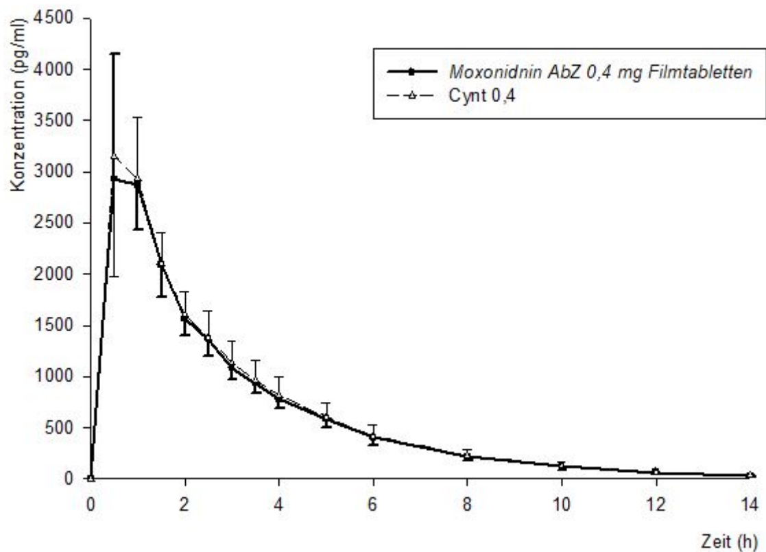
Abb. 2: Mittelwerte und Standardabweichungen der Plasmakonzentration von Moxonidin nach Einmalgabe von 1 Filmtabletten Moxonidin AbZ 0,4 mg Filmtabletten bzw. Cynt ® 0,4.
